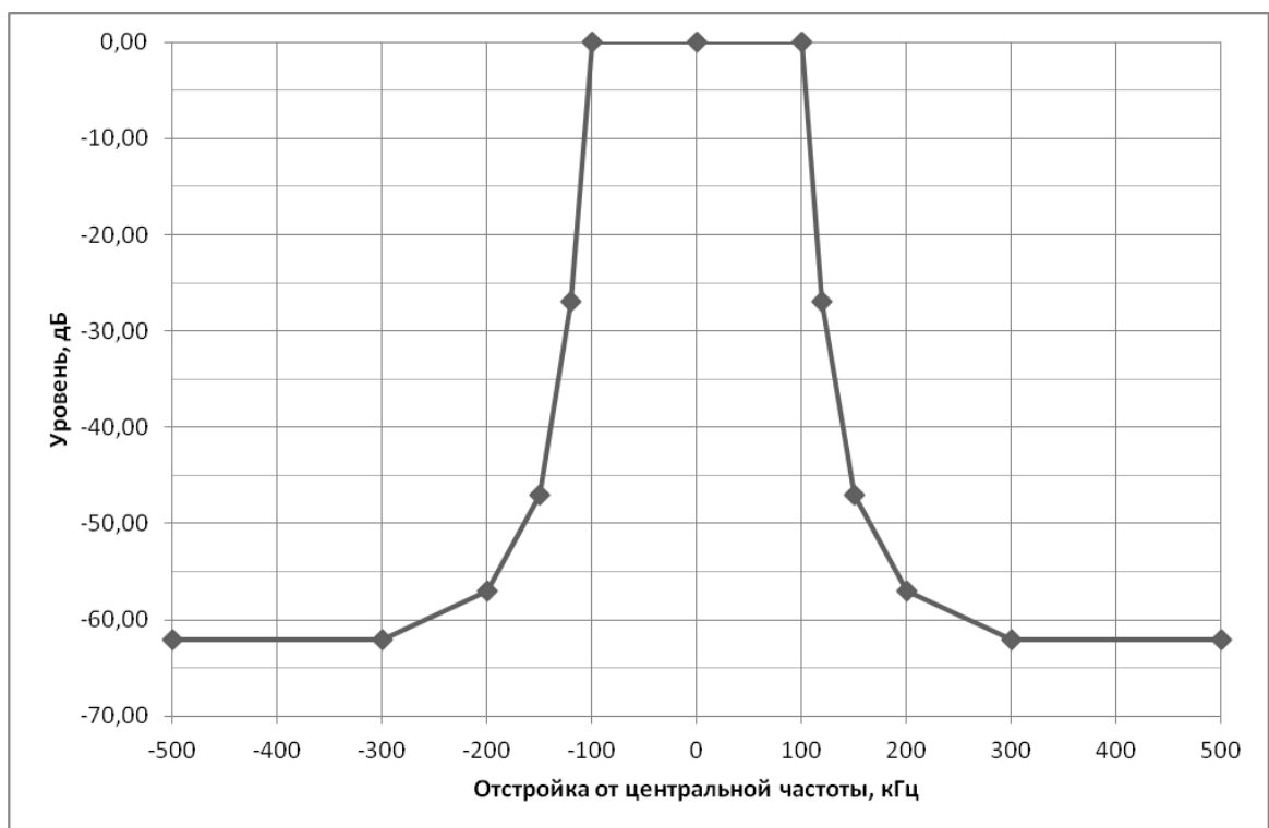
Рисунок 2 – Маска огибающей внеполосных радиоколечаний для ширины полосы частот 200 кГц
