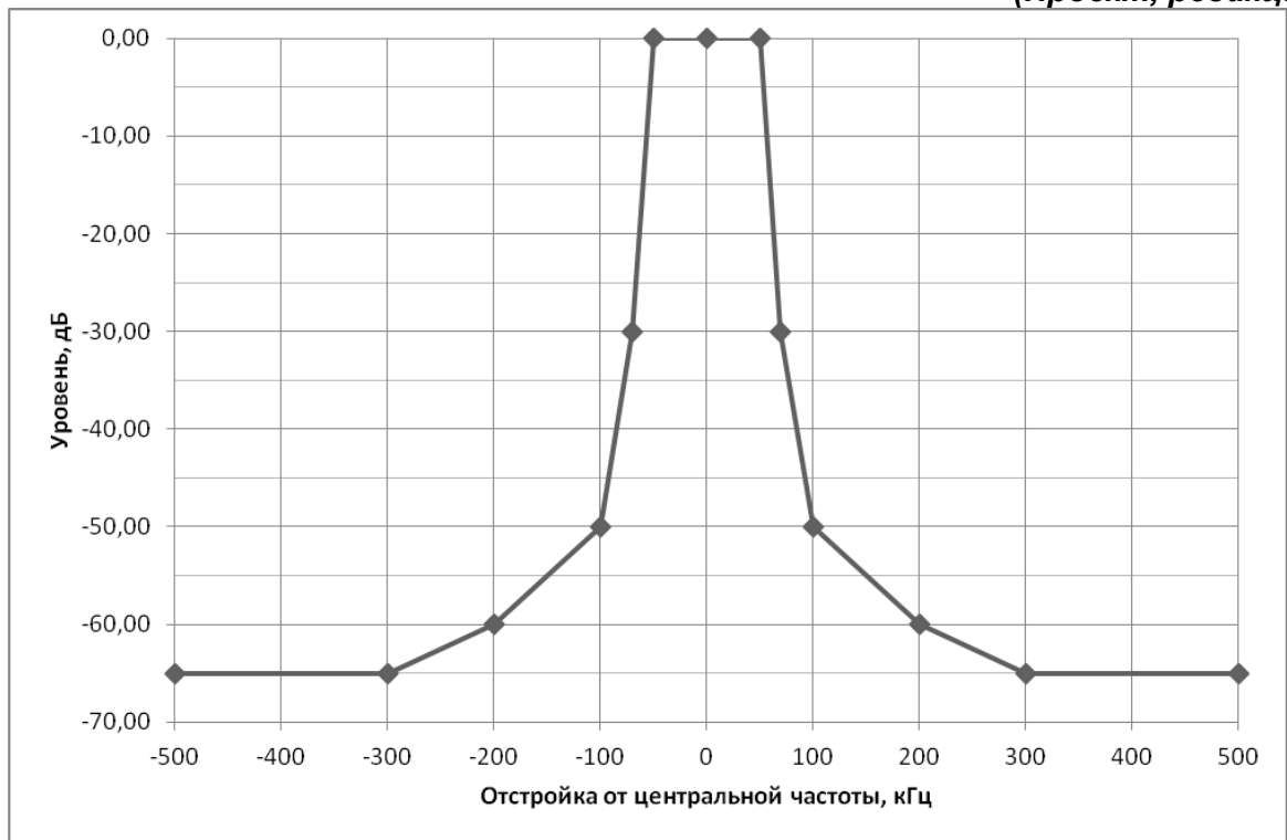
Рисунок 1 – Маска огибающей внеполосных радиоколечаний для ширины полосы частот 100 кГц
